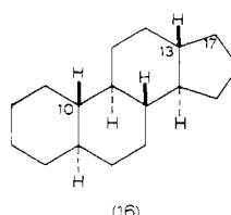
5 \alpha -Gonane
