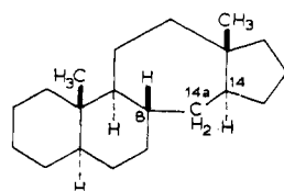
(85) C(14a) -Homo-5 \alpha -androstane
