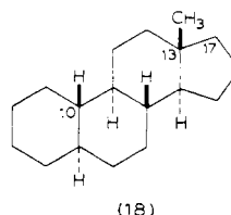
5 \alpha -Estrane
