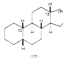
5 \beta -Gonane
